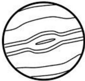
Jupiter
