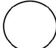
Uranus
